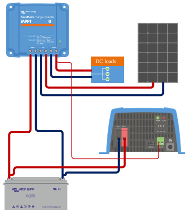
Sistemul încărcătorului solar cu invertorul conectat direct la baterie și controlat de sarcina de ieșire
