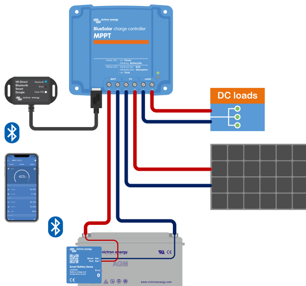
Exemplu de rețea VE.Smart Networking a unui Smart Battery Sense și a unui încărcător solar.
