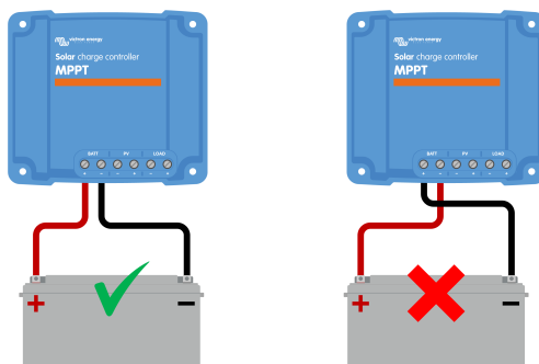
Exemple de polaritate a bateriei corectă și incorectă (inversă).
